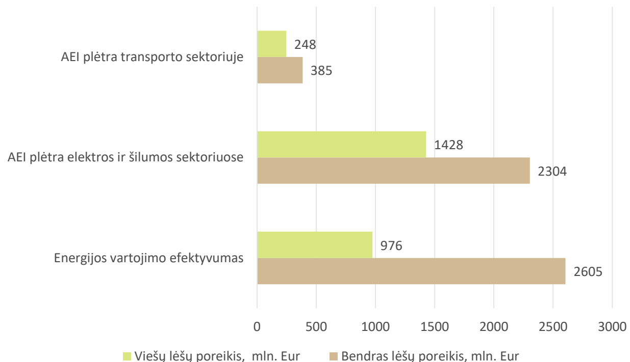
Bendras ir viešų lėšų poreikis papildomoms energetikos sektoriaus priemonėms, mln. Eur
